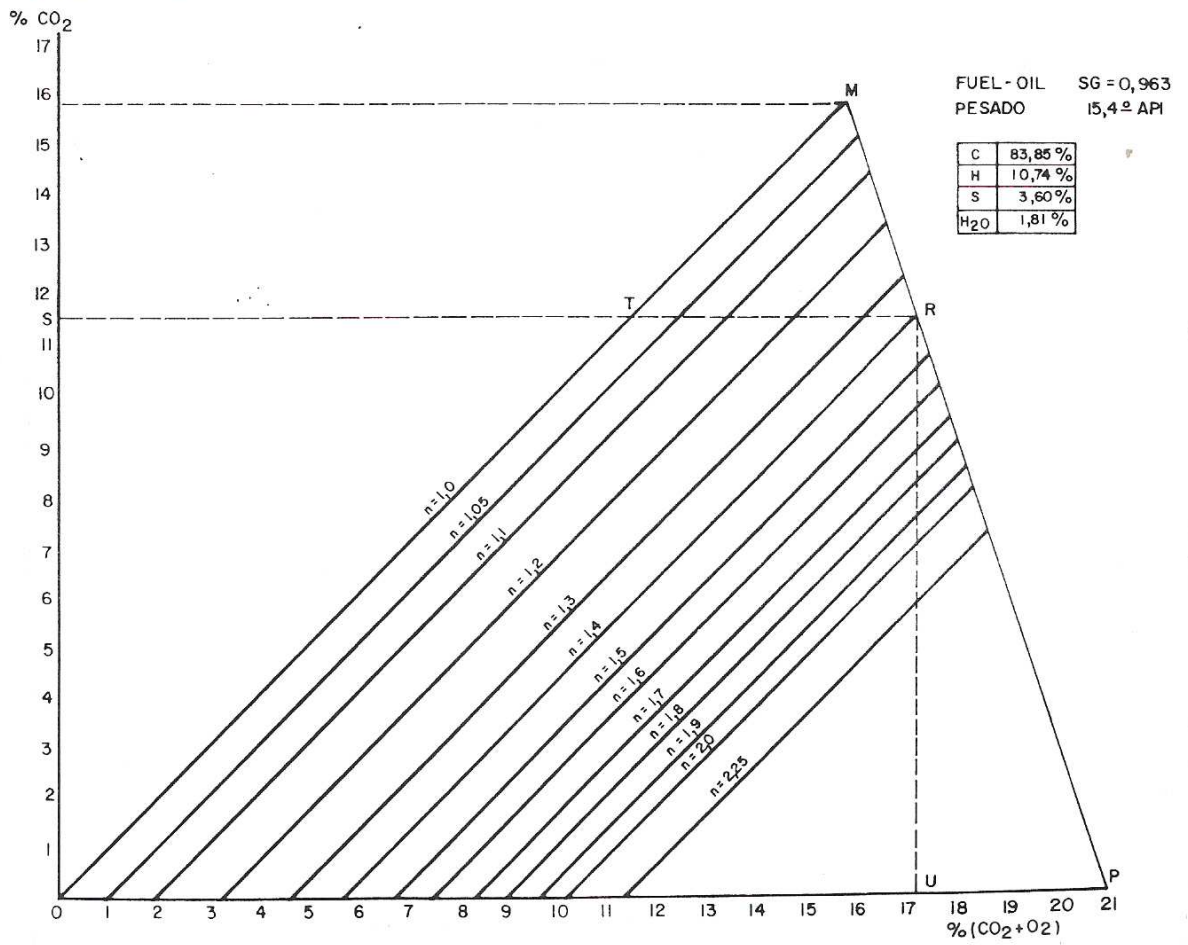
FIGURA 5.0. Diagrama de Bunte
