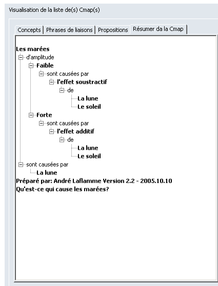
Figure 67 – Résumé « Hiérarchique ».
