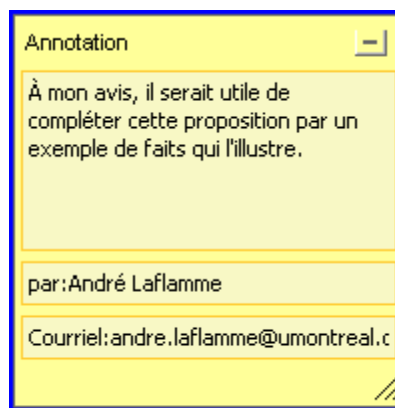
Figure 50 - Fenêtre d'annotation.
