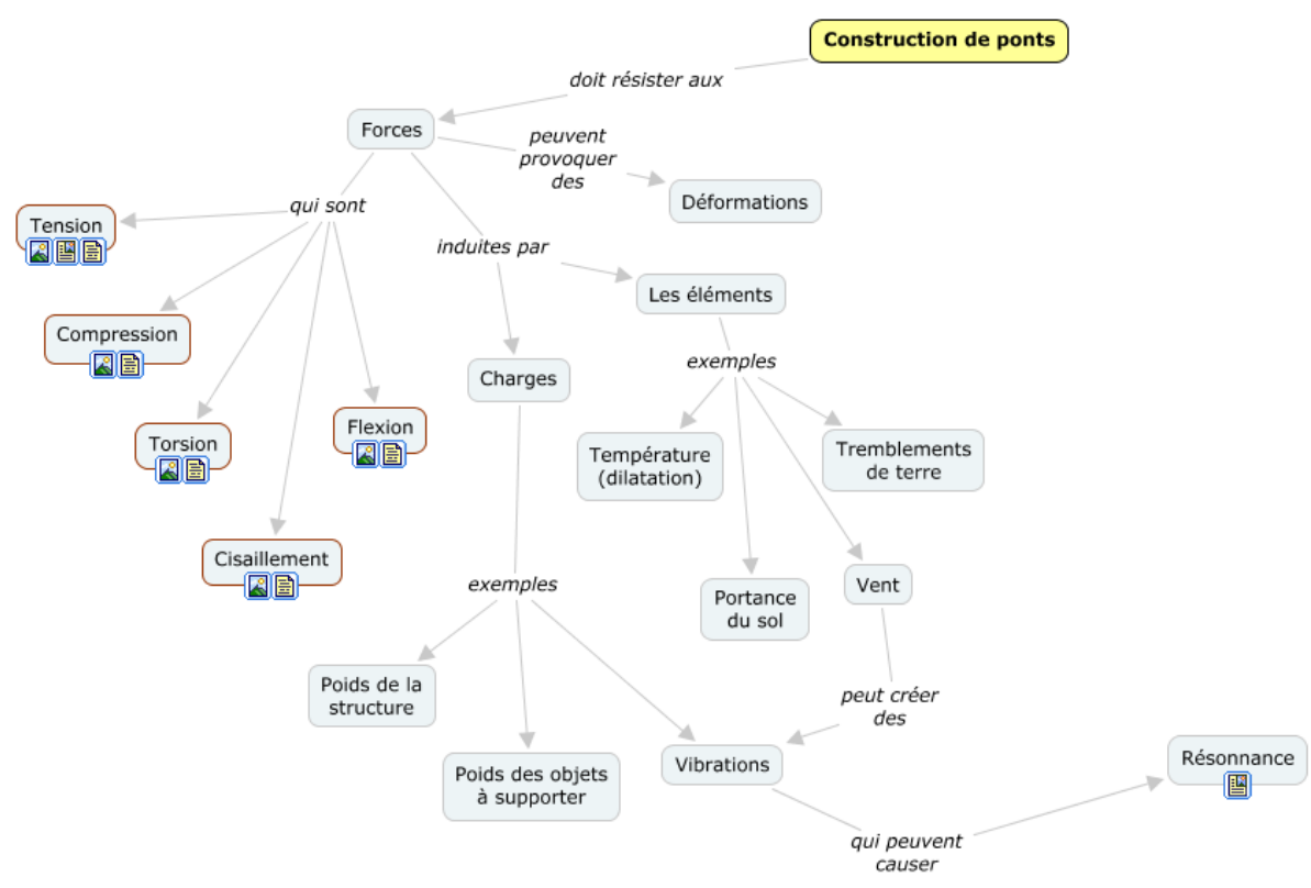
Figure 72 - Carte maitresse
