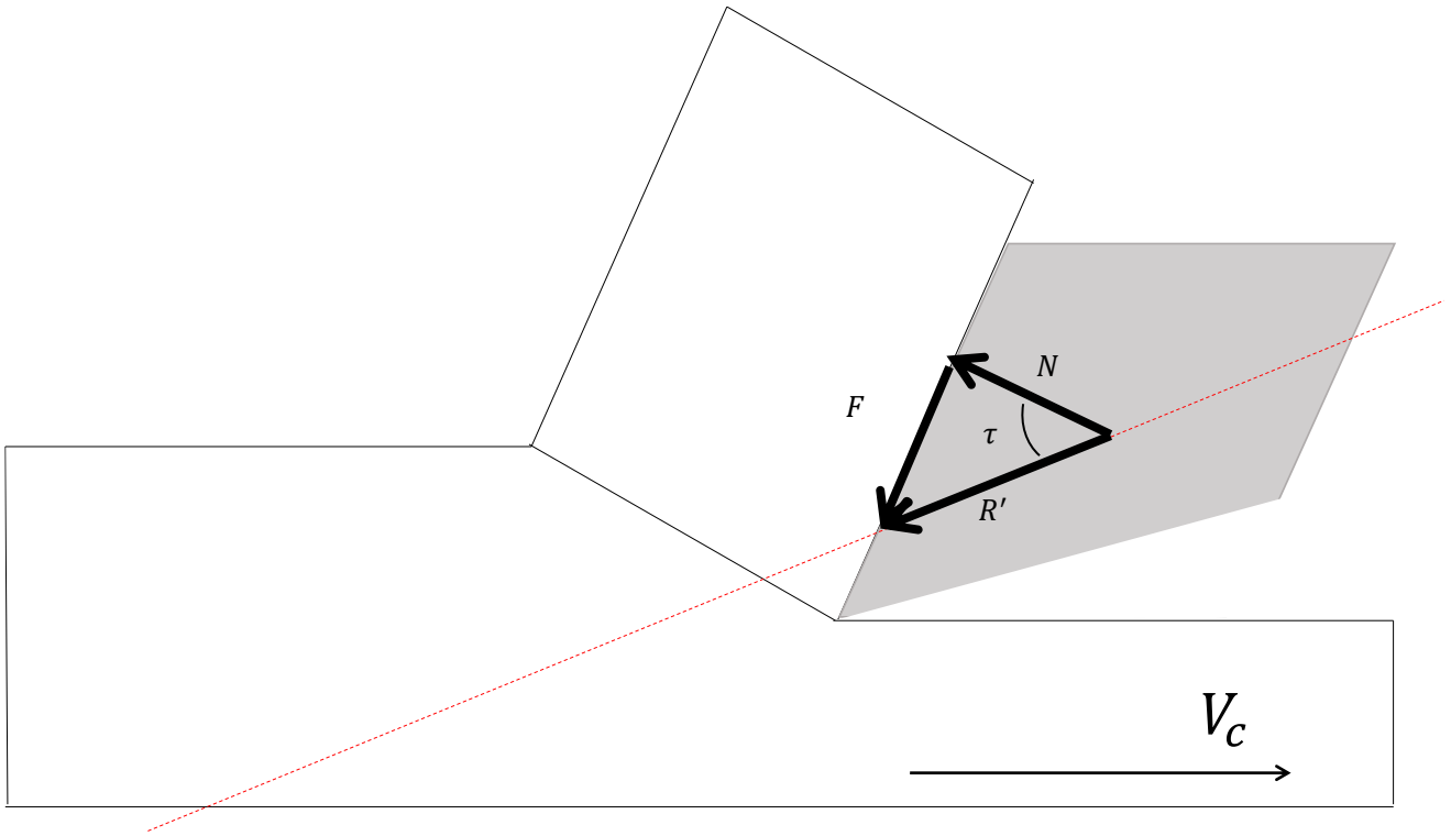
図：切削における合力 R' .
